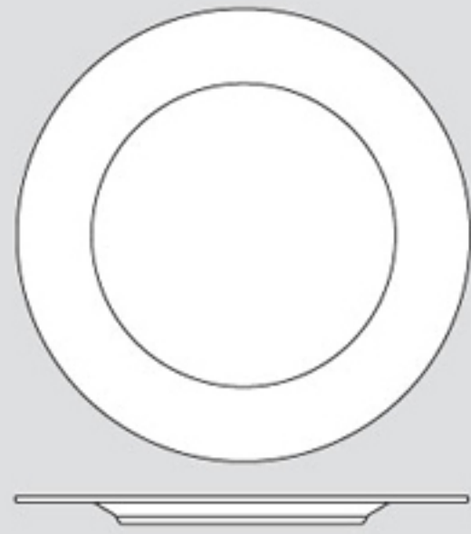
FLAT PLATE U 2202 26.0 cm. (10 1/4") 575 g. U 2203 22.5 cm. (8 7/8") 387 g. U 2204 17.0 cm. (6 3/4") 187 g.
